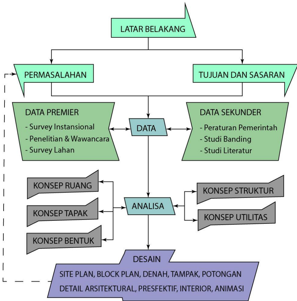
Gambar 1.1 Alur Perancangan.
