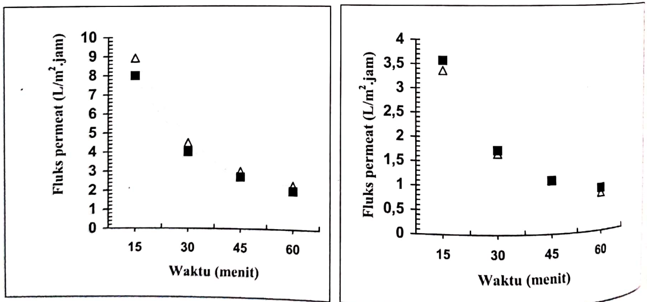
Gambar 3. Grafik hubungan fluks terhadap waktu untuk filter dengan komposisi tanah liat : abu terbang: serbuk besi = 77,5% : 20% : 2,5%, ukuran partikel abu terbang 250 \mu m dan serbuk besi a) 250 \mu m dan b) 500 \mu m (■ Laju alir umpan 7,5 L/menit, Δ Laju alir umpan 10 L/menit).
