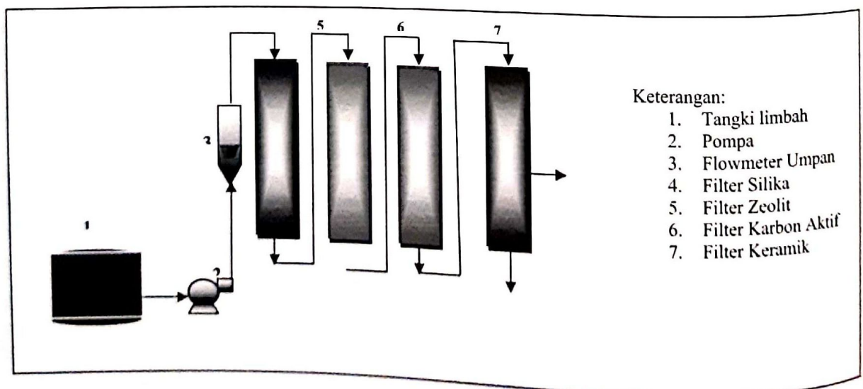
Gambar 1. Rangkaian Alat Penelitian
