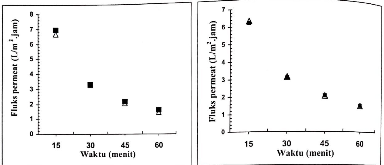
Gambar 2. Grafik hubungan fluks terhadap waktu untuk filter dengan komposisi tanah liat : abu terbang: serbuk besi = 80% : 20% : 0%, ukuran partikel abu terbang 250 \mu m dan serbuk besi a) 250 \mu m dan b) 500 \mu m (■ Laju alir umpan 7,5 L/menit, Δ Laju alir umpan 10 L/menit)
