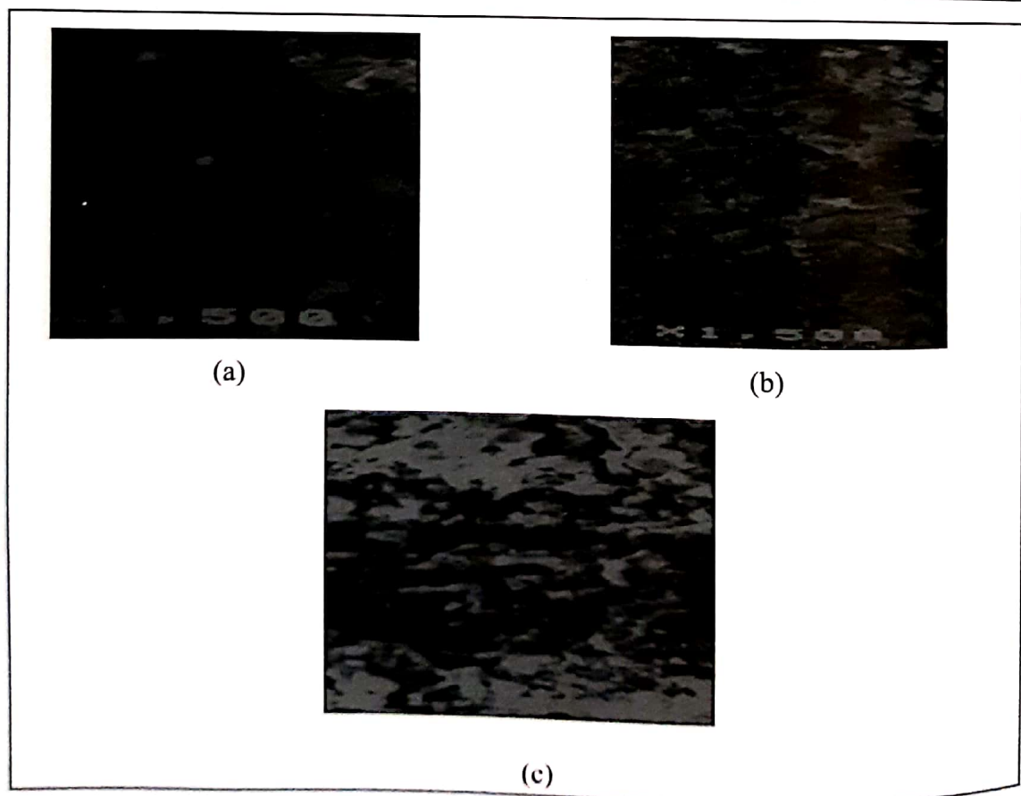
Gambar 4. Citra SEM untuk filter dengan komposisi tanah liat : abu terbang : serbuk besi 67,5%:2,5%:7,5% dengan ukuran partikel abu terbang serta serbuk besi 250 \mu m yang diperbesar 1500 kali (a) bagian inlet filter, (b) bagian tengah filter, dan (c) bagian outlet filter.
