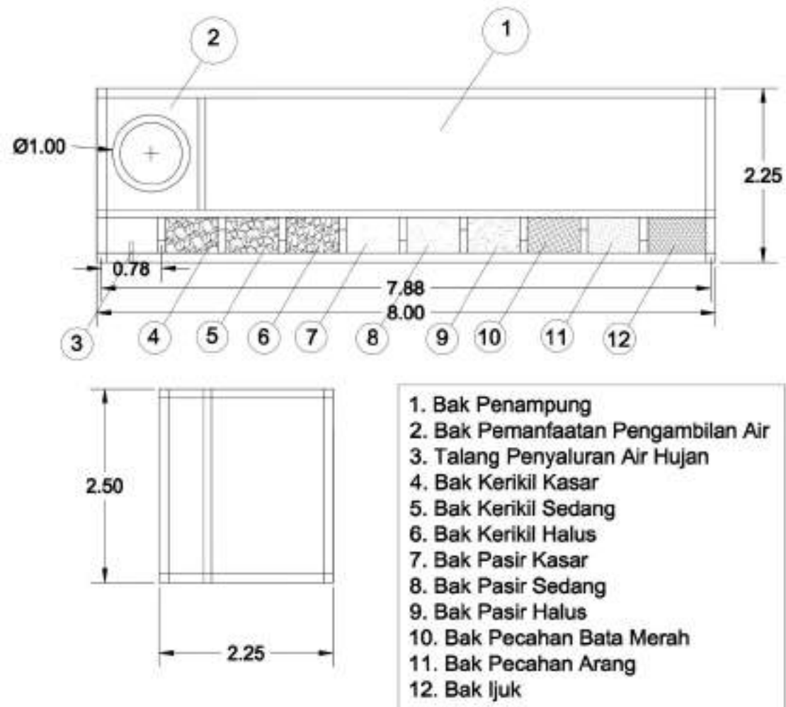
Gambar Perencanaan Bak Akuifer Buatan (ABSAB)
