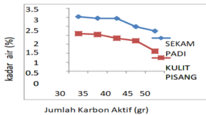
Gambar 1. Grafik massa karbon aktif terhadap kadar air
