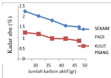
Gambar 2. Grafik jumlah adsorben terhadap kadar abu
