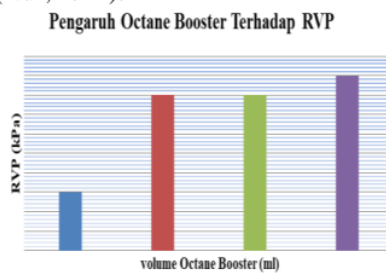
Gambar 3. Grafik Pengaruh Penambahan Octane Booster Terhadap RVP
