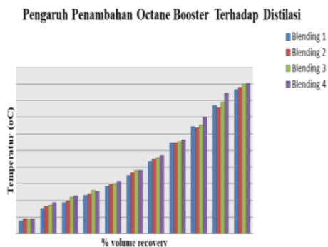
Gambar 2. Grafik Pengaruh Penambahan Octane Booster Terhadap Distilasi
