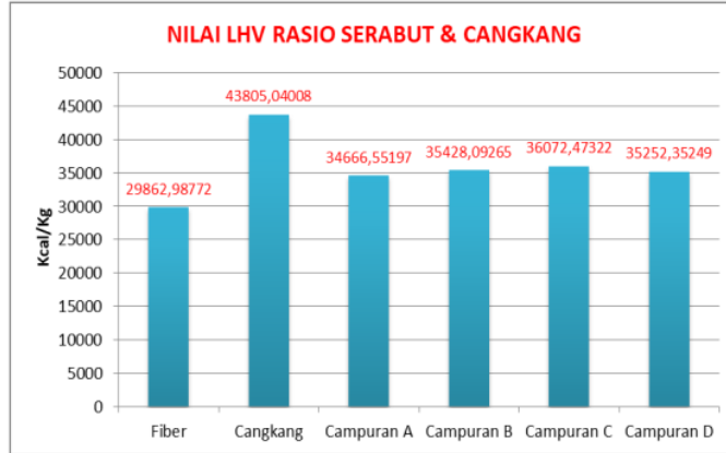
Gambar 2. Grafik perbandingan nilai LHV Rasio Serabut & Cangkang
