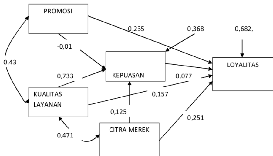
Gambar 3. Diagram Jalur Lengkap Penghitungan Pengaruh
