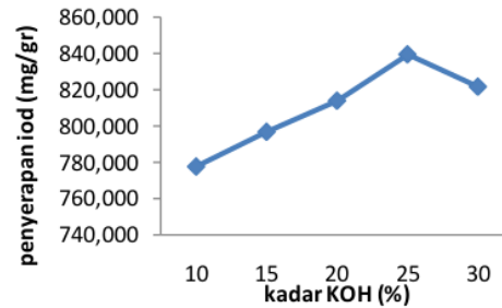
Gambar 3. Pengaruh Konsentrasi KOH terhadap Penyerapan Iod
