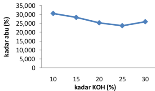
Gambar 2. Pengaruh Konsentrasi KOH terhadap Kadar Abu
