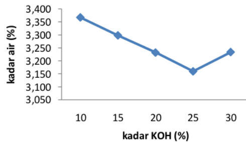
Gambar 1. Grafik Pengaruh Konsentrasi KOH terhadap Kadar Air
