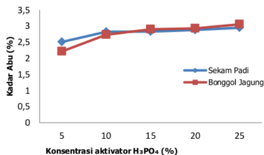
8 Gambar 2. Grafik hubungan antara konsentrasi aktivator H 3 PO 4 terhadap kadar abu karbon aktif
