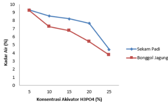
9 4 Gambar 1. Grafik hubungan antara konsentrasi aktivator H 3 PO 4 terhadap kadar air karbon aktif
