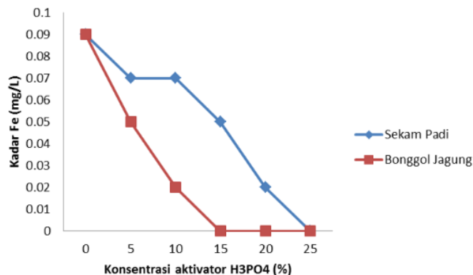
Gambar 8. Grafik hubungan Kandungan besi dengan konsentrasi aktivator
