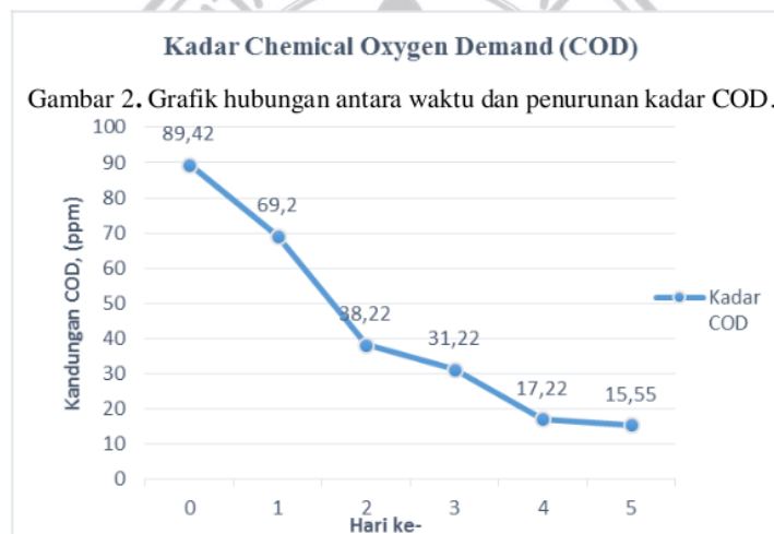
Gambar 2. Grafik hubungan antara waktu dan penurunan kadar COD.
